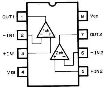
● BA728/NJM2904D (OP Amp.)
